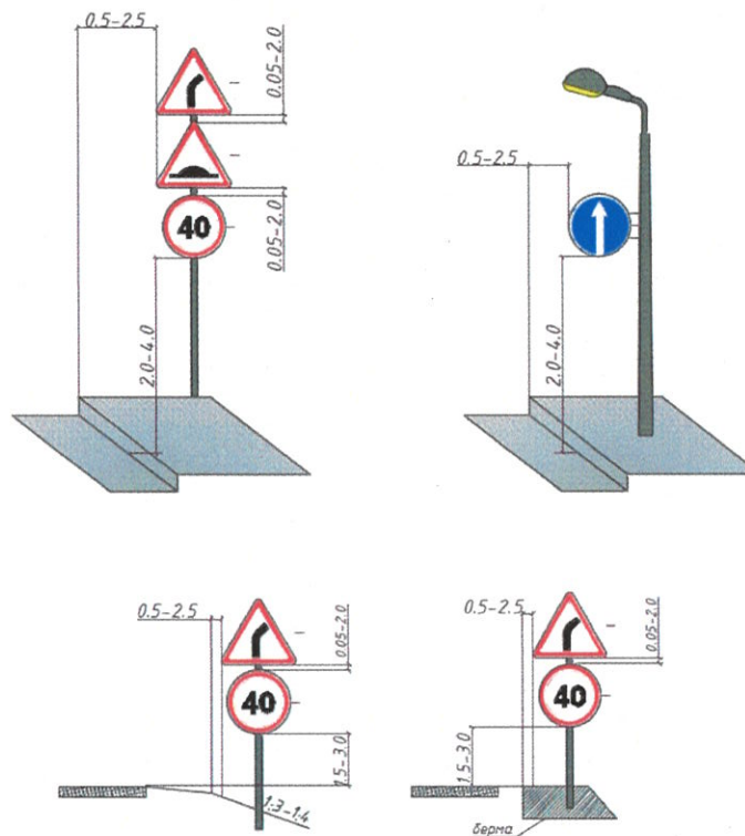
Рисунок 3 – Способы установки дорожных знаков
